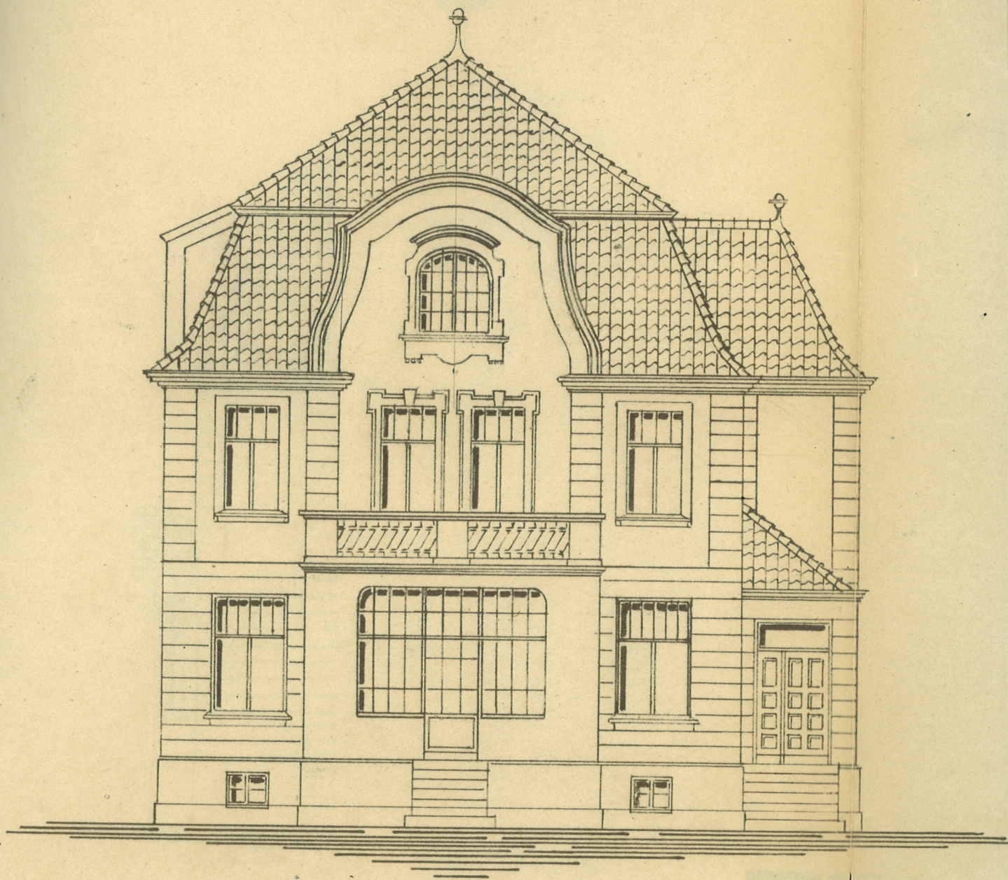
VORDER ANSICHT
