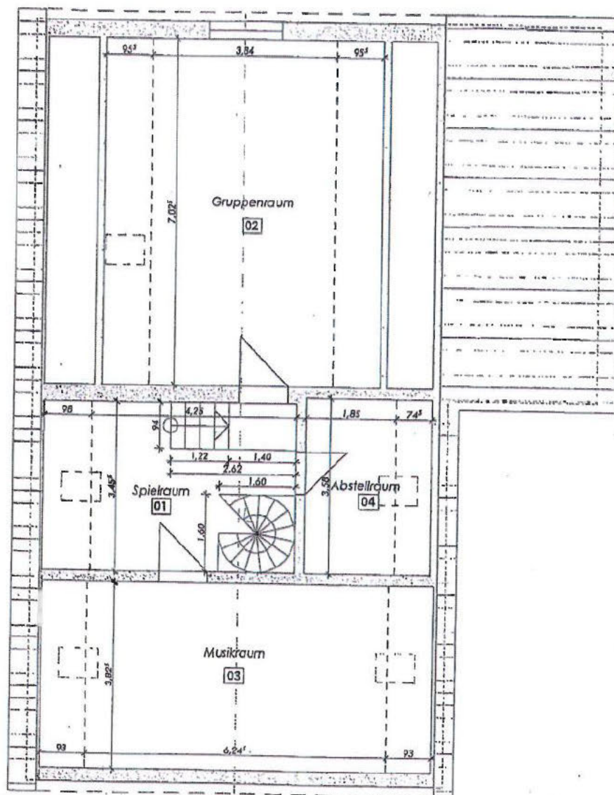
Dachgeschoss
