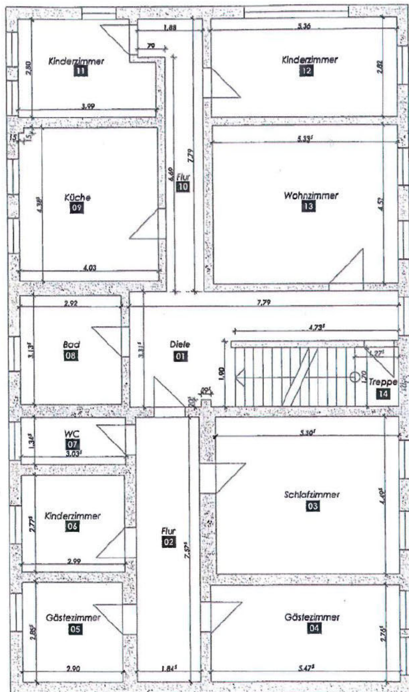
Obergeschoss
