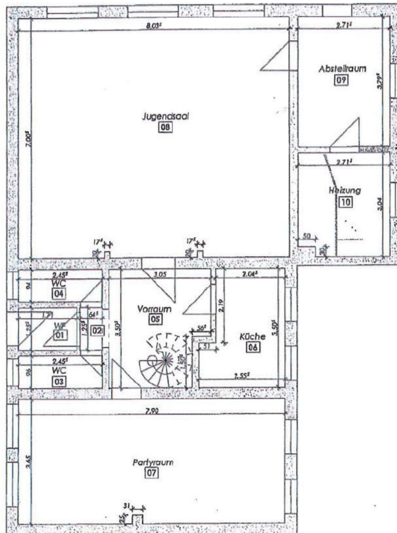
Erdgeschoss
