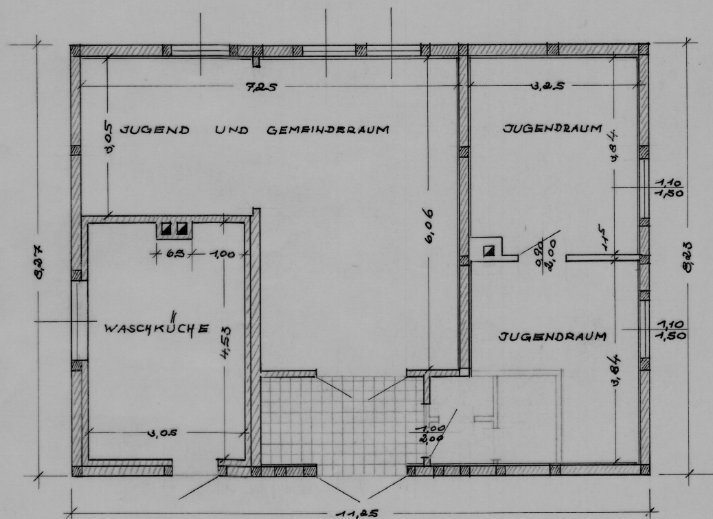
ERDGESCHOSS
