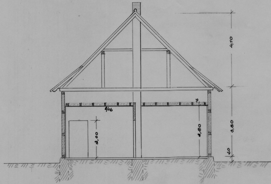
SCHNITT A-B
