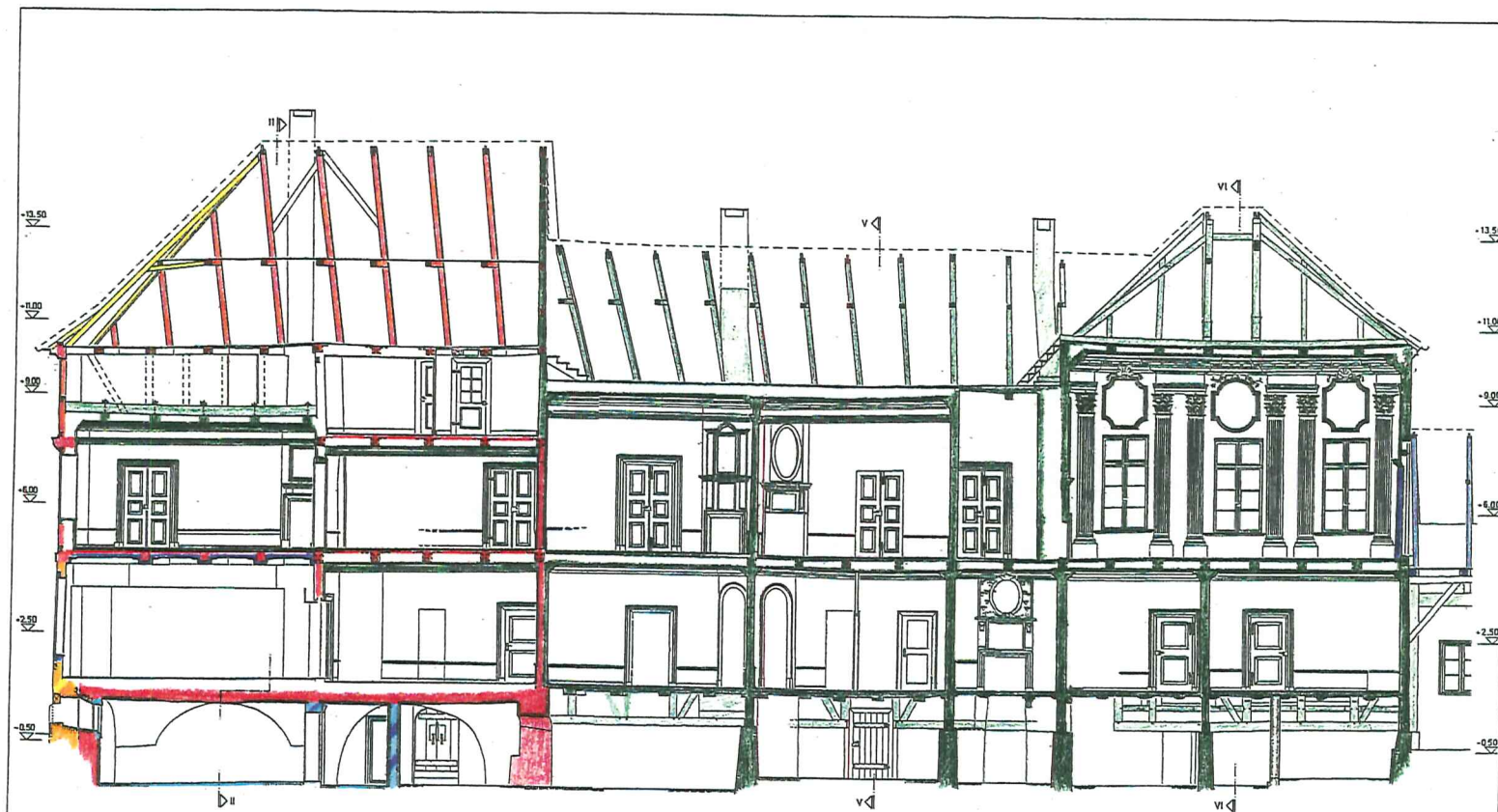
LÄNGSSCHNITT IV-IV SEITENFLÜGEL
