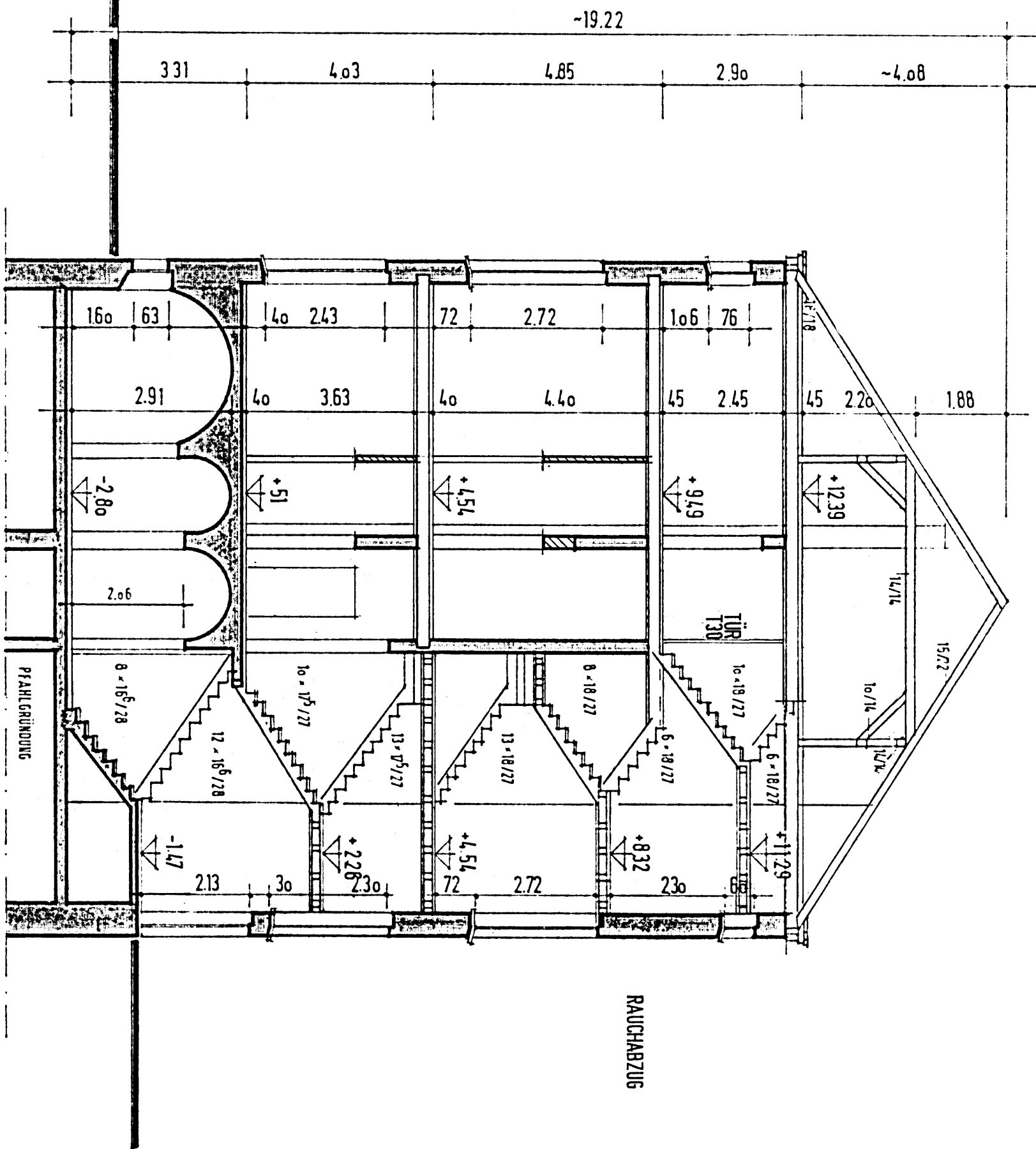
SCHNITT E-F
