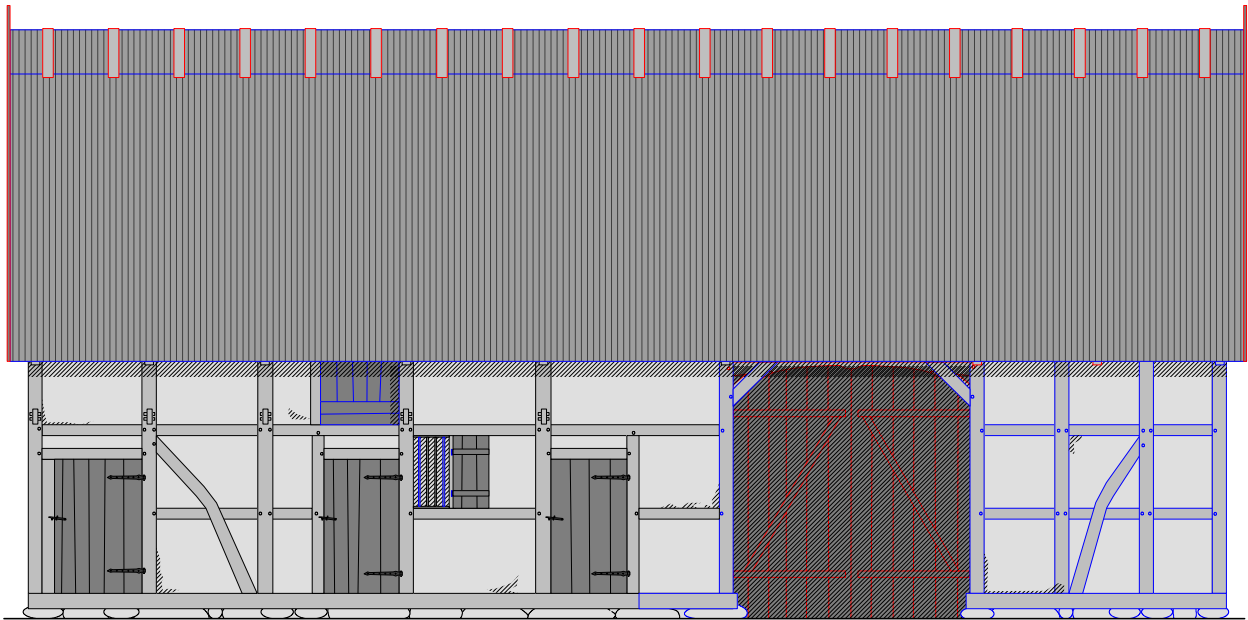
Traufseite West, bauzeitlicher Zustand 1815
