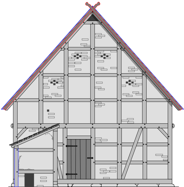
Giebel Nord, Umbauzustand um 1950
