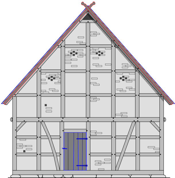
Giebel Nord, bauzeitlicher Zustand 1815
