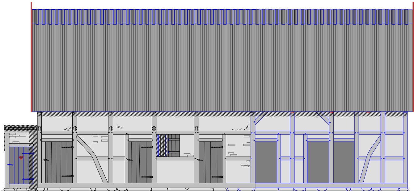
Traufseite West, Umbauzustand um 1950
