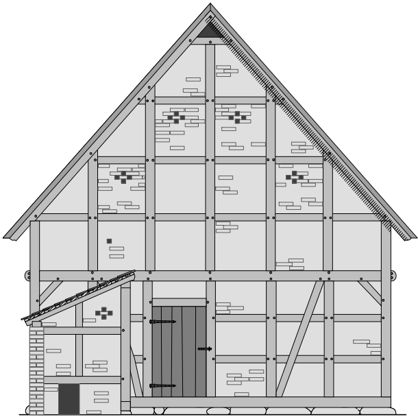
Giebel Nord, Zustand 2019
