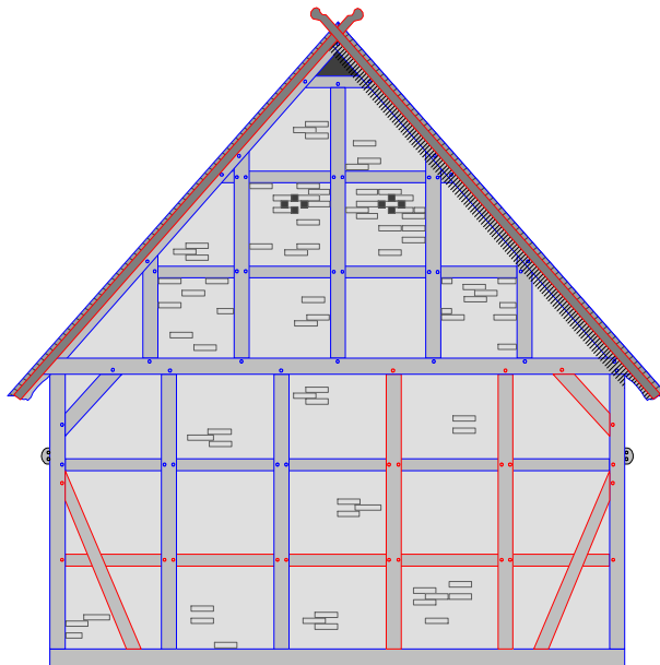
Giebel Süd
