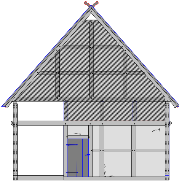
Querwand von Nord
