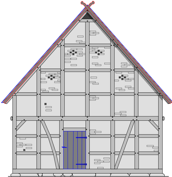
Giebel Nord
