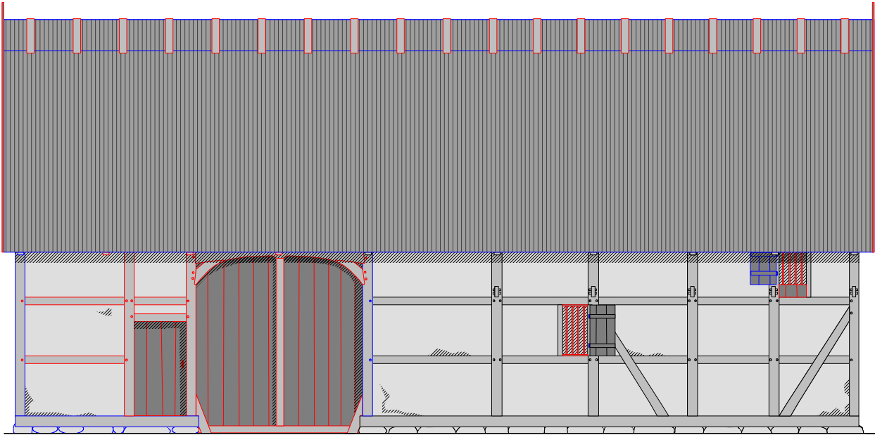
Traufseite Ost; mit Toreinfahrt
