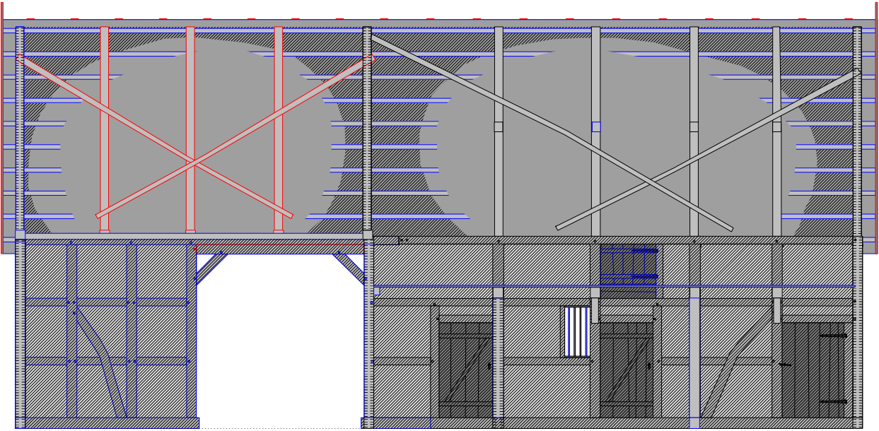
Längsschnitt, Westtraufe innen
