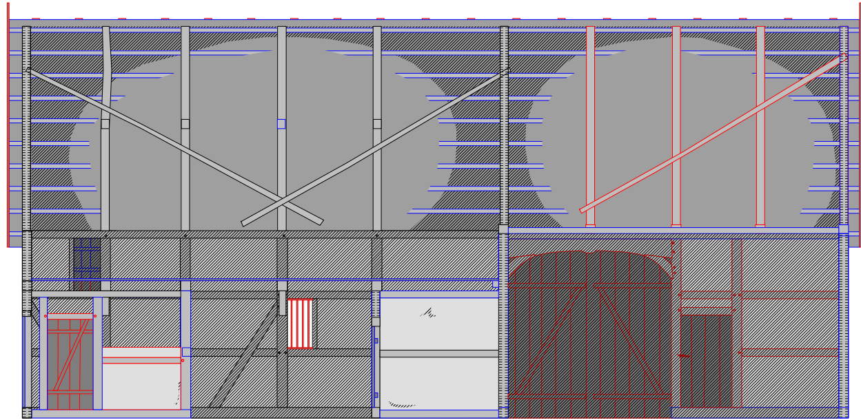
Längsschnitt, Osttraufe innen
