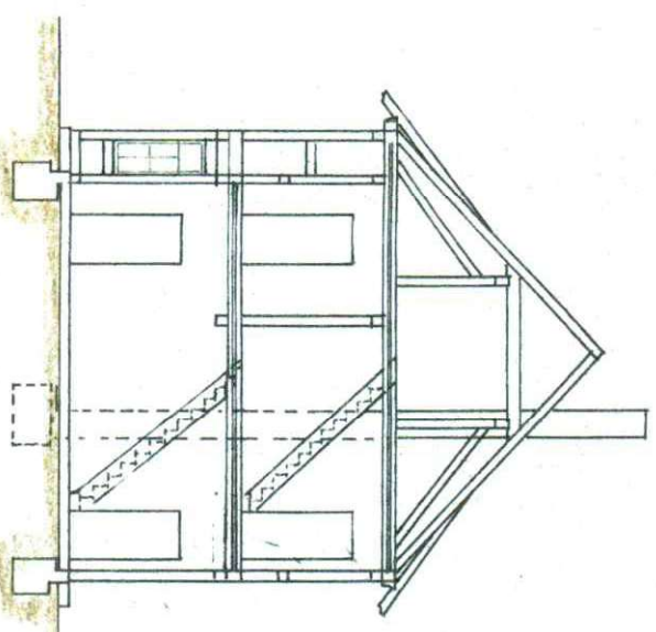
Querschnitt.
