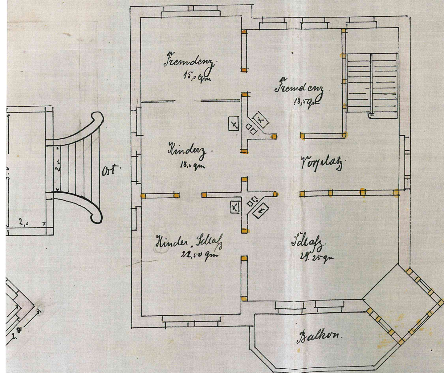
1 er Étage.
