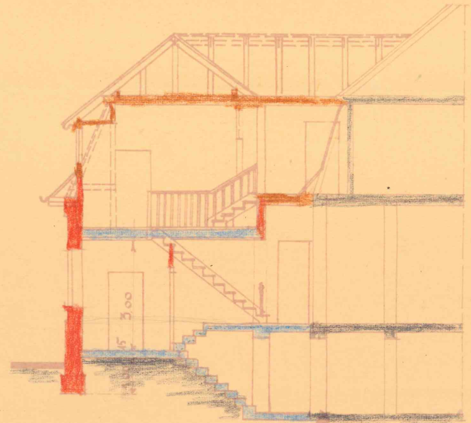
SCHNITT A-B
