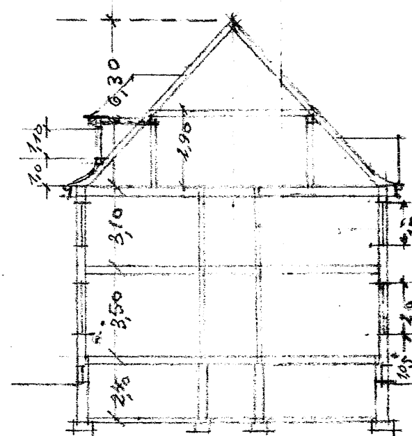
Schnitt a-b.
