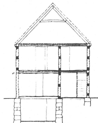
SCHNITT A - A
