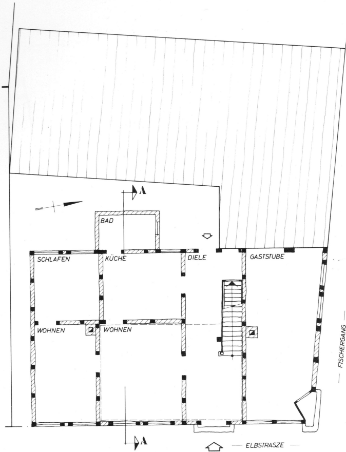
UNTERSTOCK
