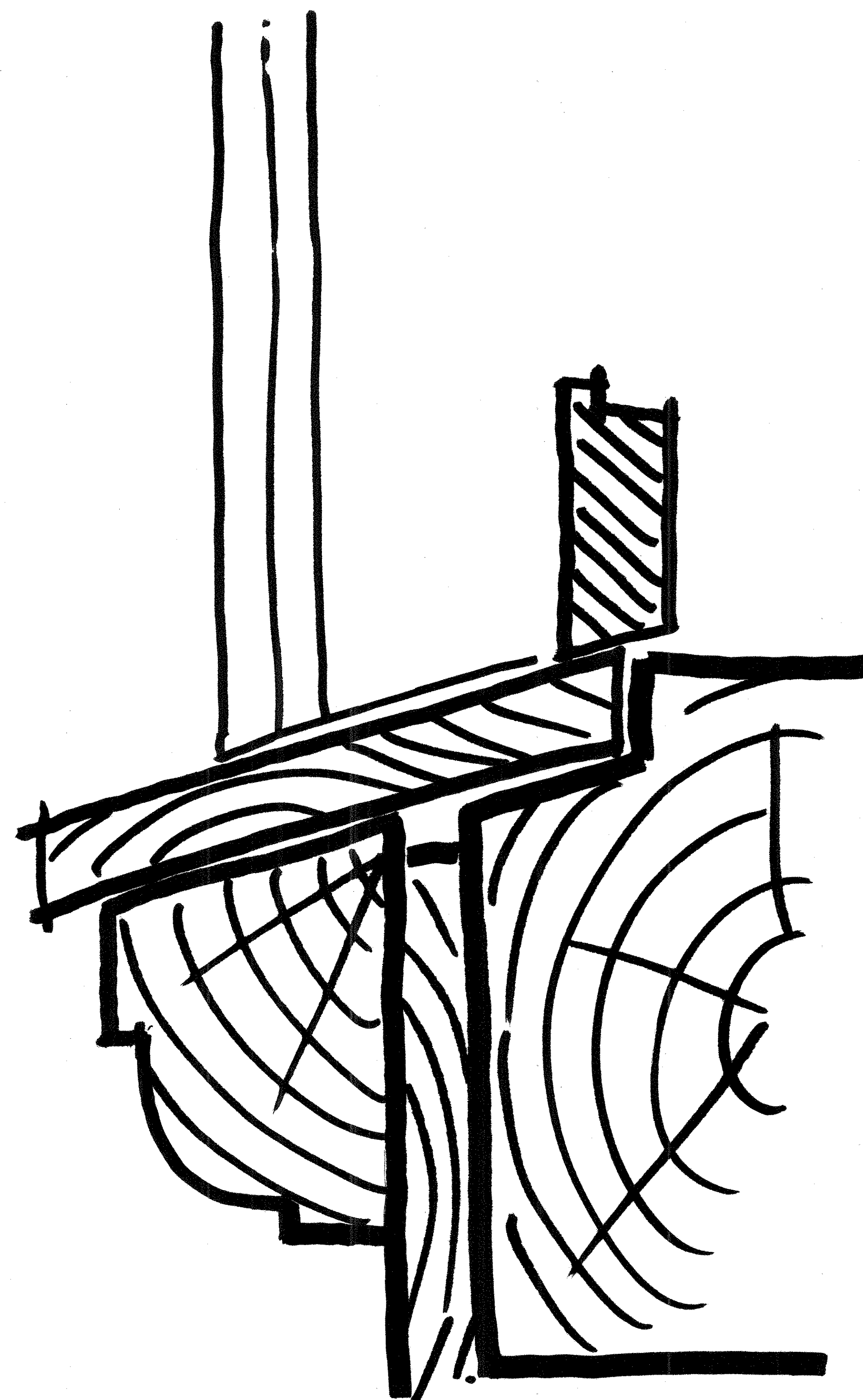
FENSTERBRÜSTUNG
