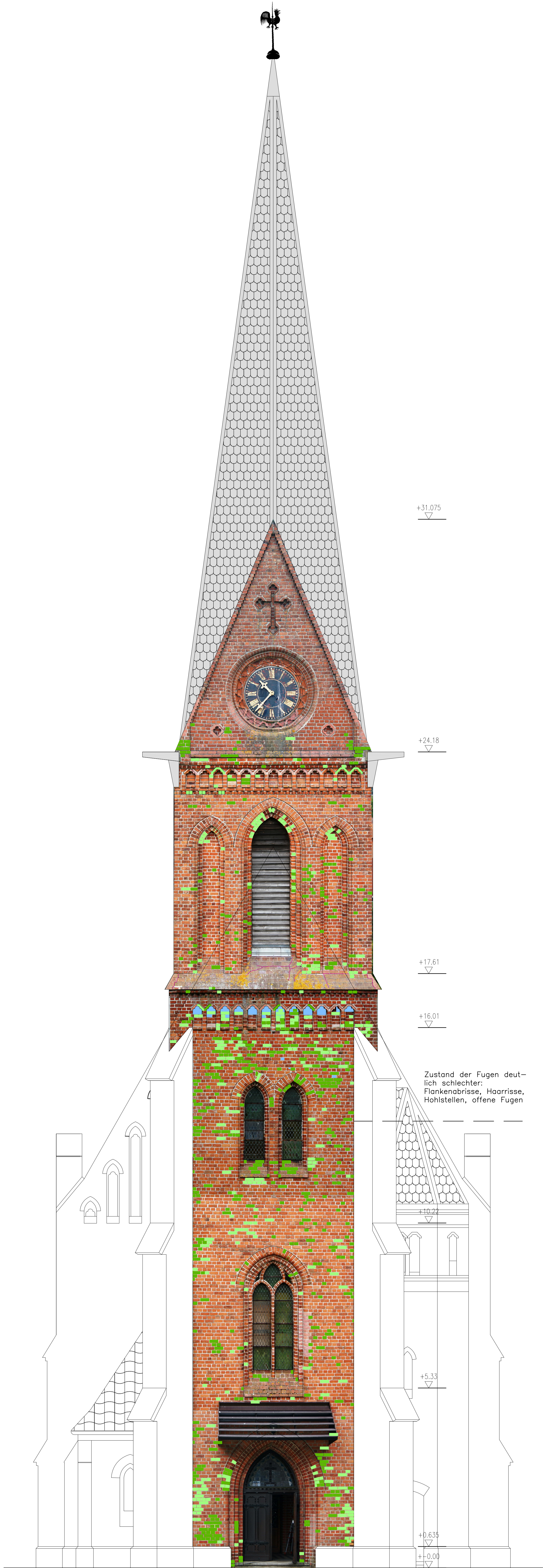
ANSICHT P (WESTANSICHT)
